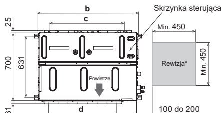
Wylot powietrza
