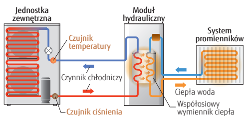
Typ Split
