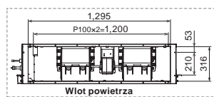
Model: ARXC036/ARXC045/ARXC060
