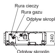
Odpływ skroplin
